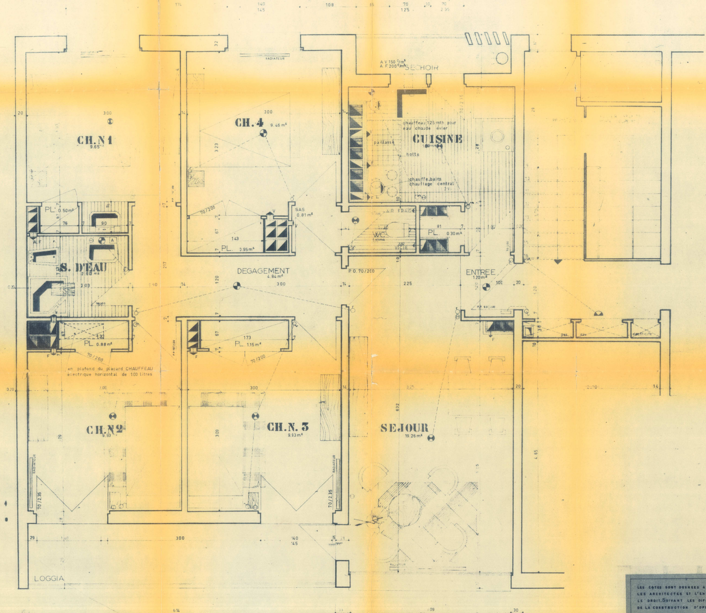
DETAIL DE L'ENSEMBLE POUR LE BATIMENT F5
